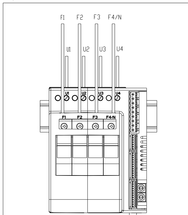
Figura 11 modello con portafusibili
