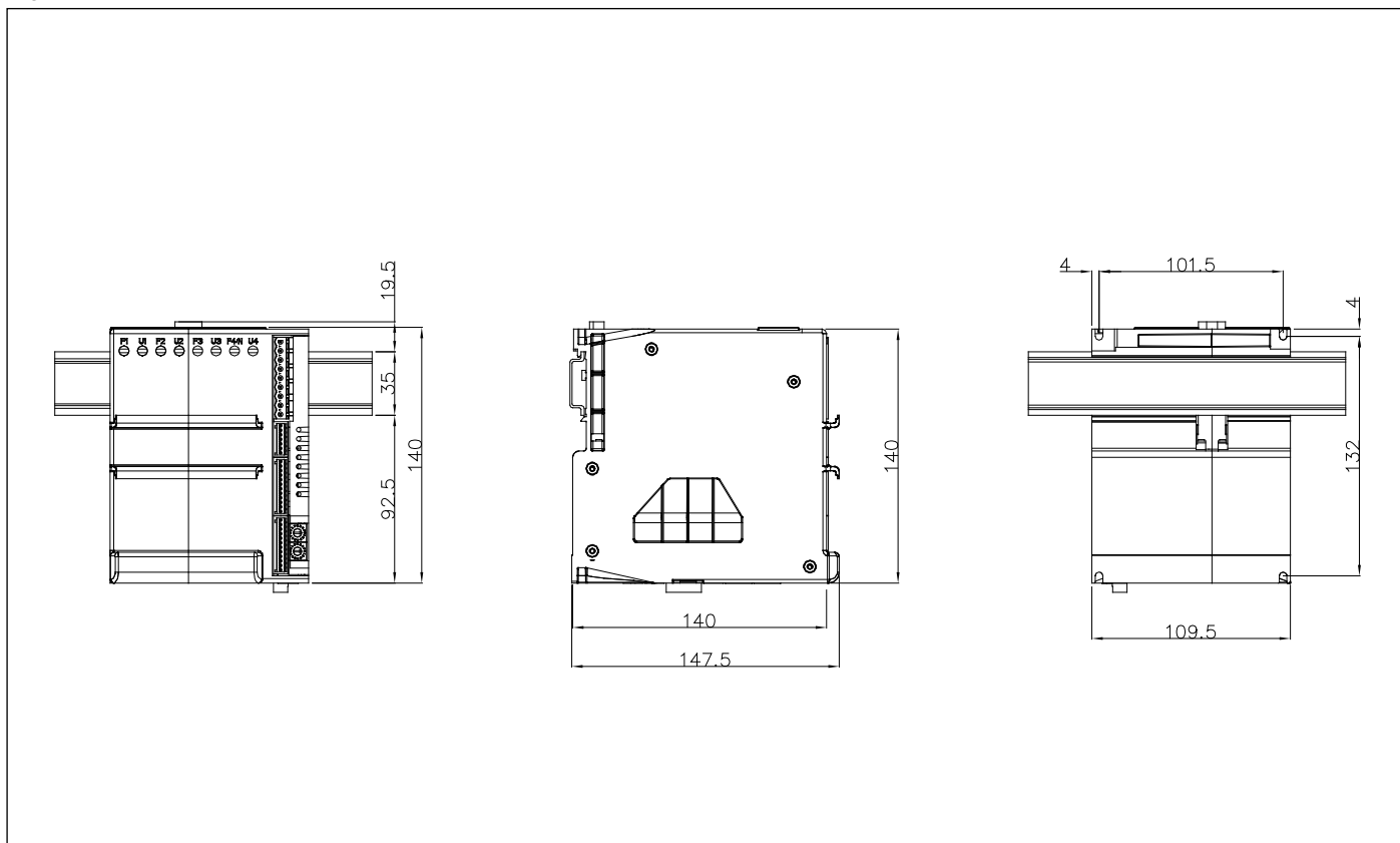
Figura 4 Modello senza portafusibili
