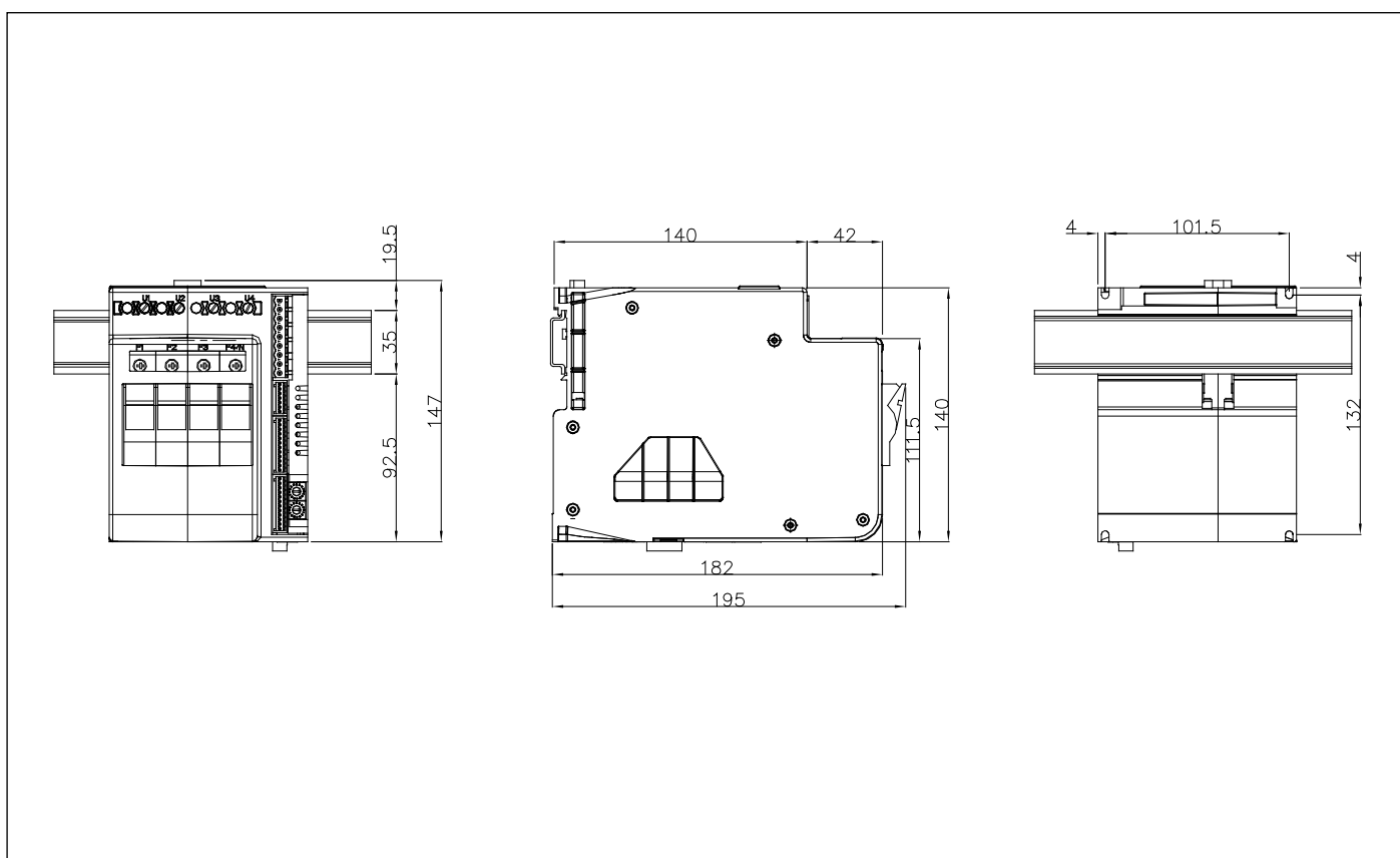
Figura 5 Modello con portafusibili
