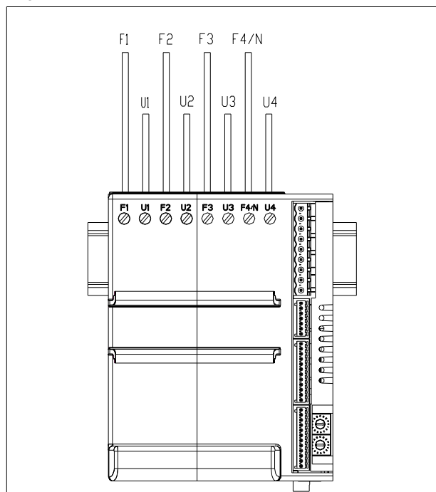
Figura 10 modello senza portafusibili
